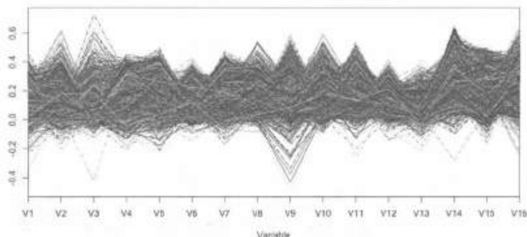
图 4.6 随机森林拟合例4.1数字笔迹识别数据的局部变量重要性图
