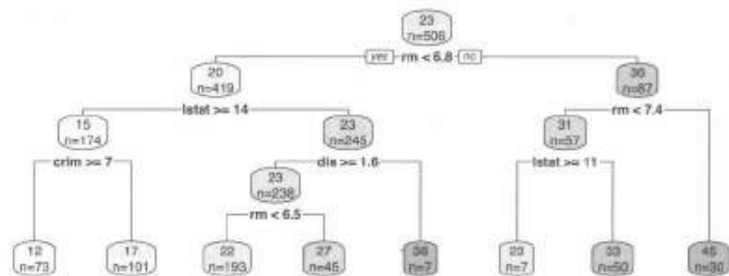
图 3.9 对例3.1波士顿住房数据做决策树回归的结果
