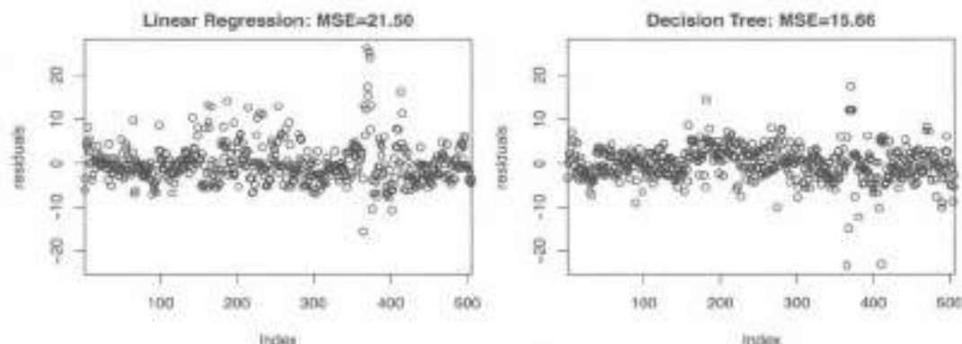
图 3.10 例 3.1 波士顿房价数据的线性回归 (左) 和决策树回归的残差图 (右)
