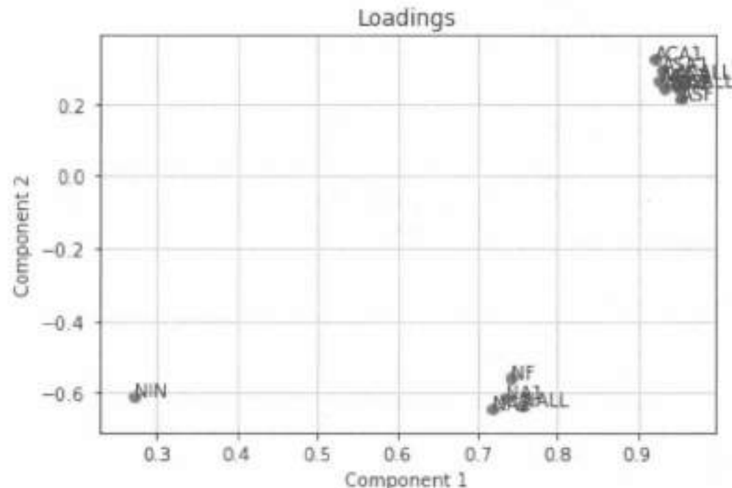
图 5.15 例5.1教师数据主成分分析的载荷图
