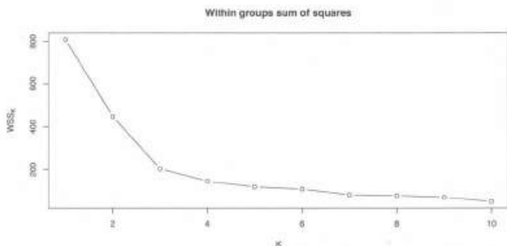
图 7.12 例 7.4 人造数据用不同的 k 所得到的类内平方和
