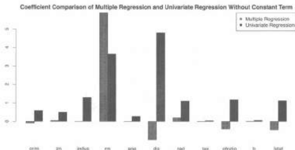
图 3.6 对例3.1的波士顿住房数据去掉变量 chas 和 nox 后每个自变量的简单回归和多重回归系数估计的变化
