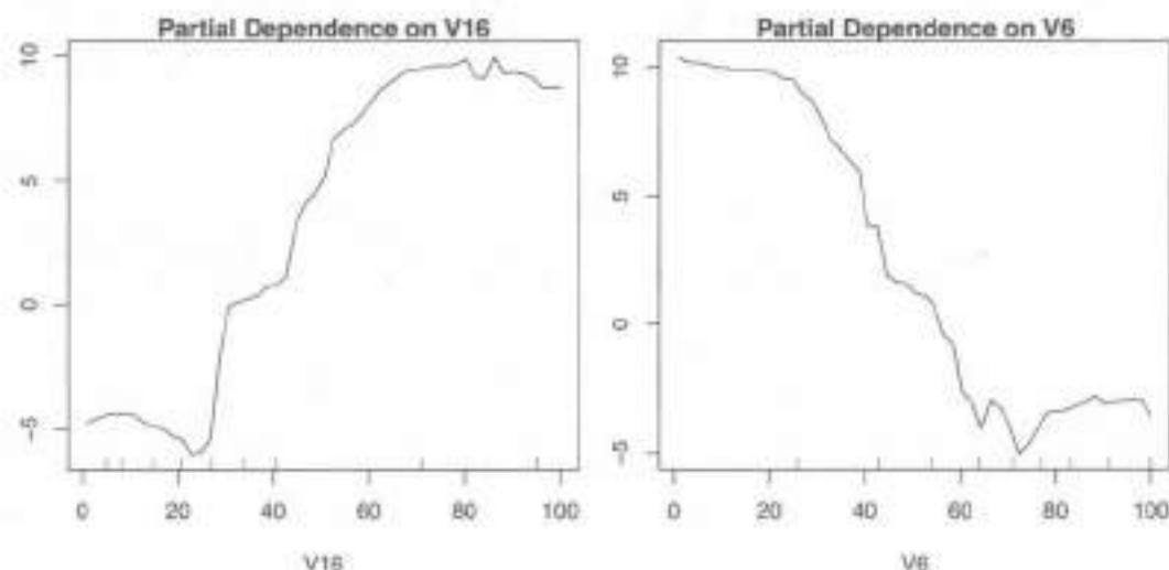
图 4.7 随机森林拟合例4.1数字笔迹识别数据对 2 个变量的部分依赖性图
