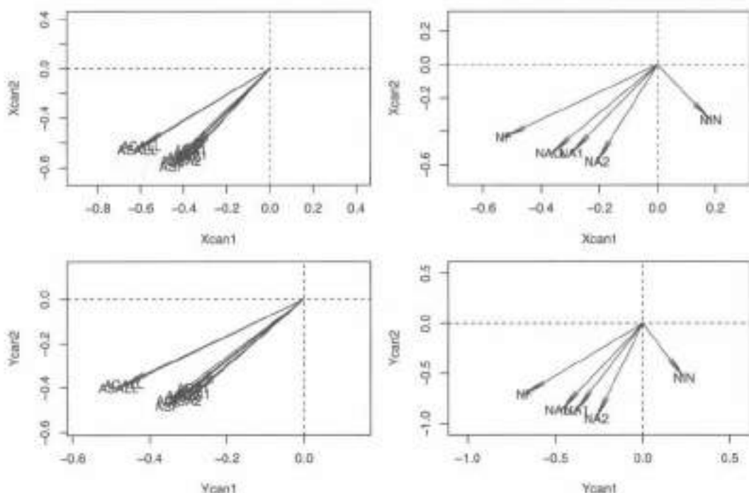
图 8.8 例 8.1 教师数据在第一、二个典型变量坐标中显示四组相关的情况
