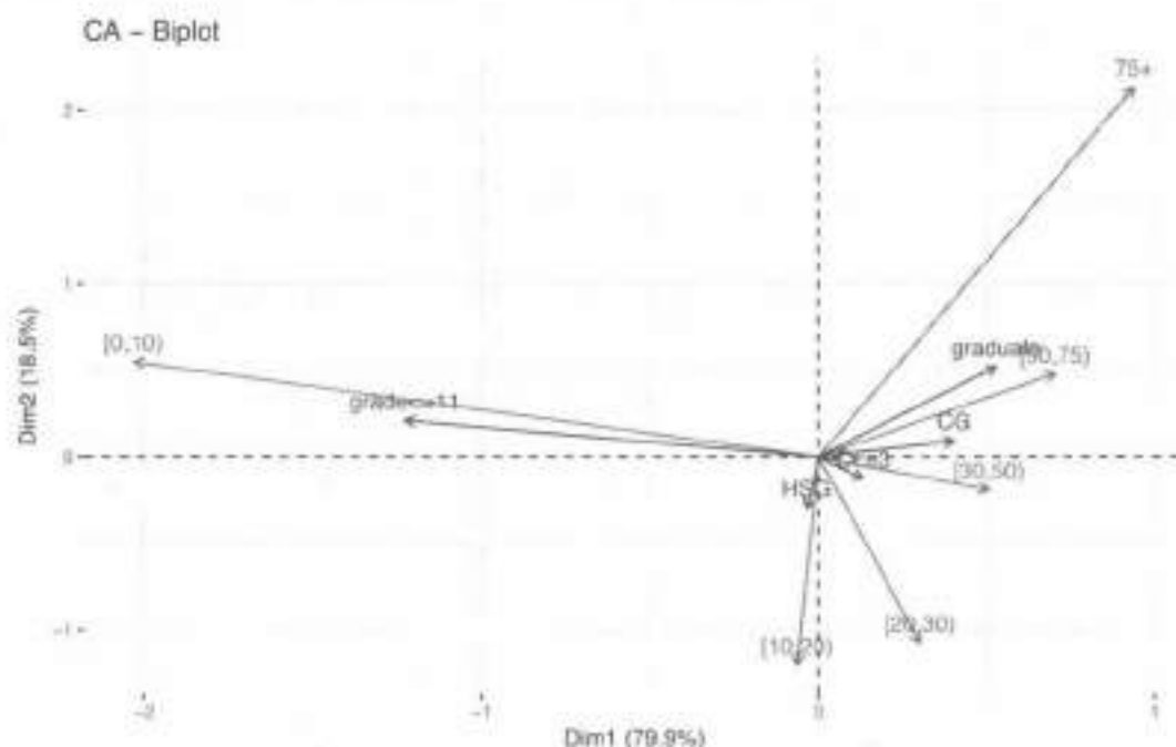
图 9.2 例9.1收入数据的收入和教育列联表的对应分析结果
