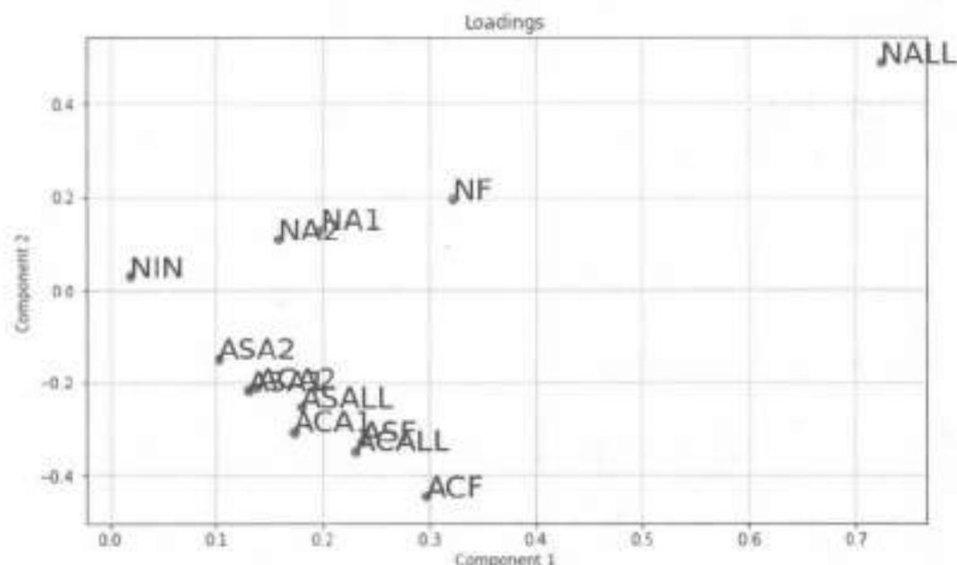
图 5.17 例5.1教师数据主成分分析的载荷图
