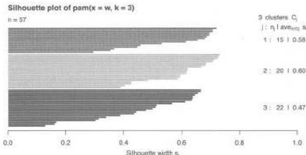
图 7.20 对例7.4人造数据展示每个观测值的轮廓宽度
