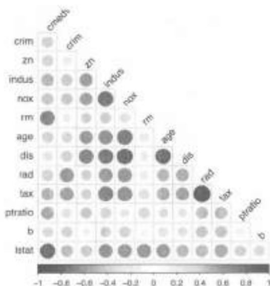
图 3.4 例3.1波士顿住房数据变量的线性相关系数展示
