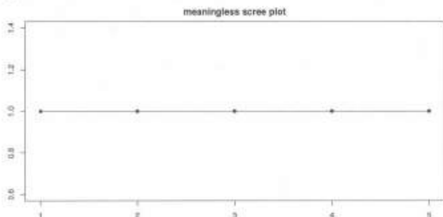
图 5.5 没有意义的主成分分析的崖底碎石图
