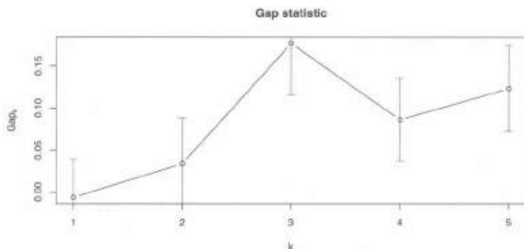
图 7.19 对例7.4人造数据使用 Gap 统计量来确定聚类数目
