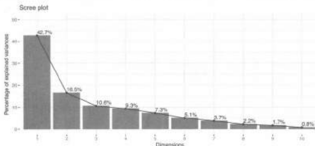
图 5.10 例5.3主成分分析的崖底碎石图
