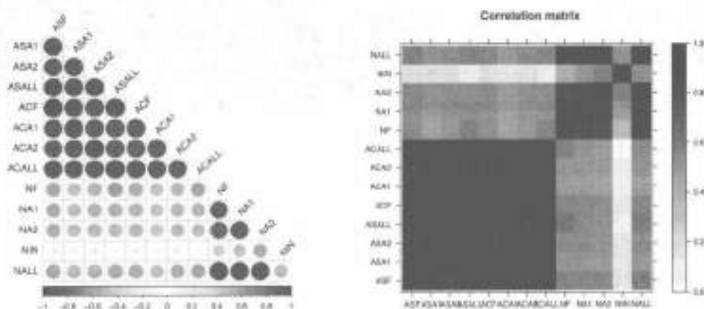
图 5.1 例5.1数据数据的线性相关系数两种直观展示
