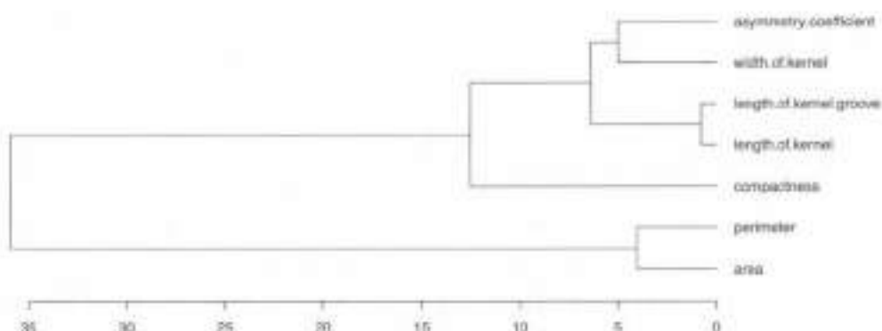
图 7.29 例7.6种子数据对变量分层聚类的树状图
