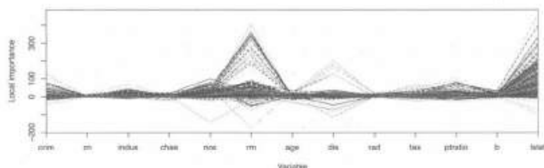
图 3.13 随机森林拟合例3.1波士顿房价数据的局部变量重要性图
