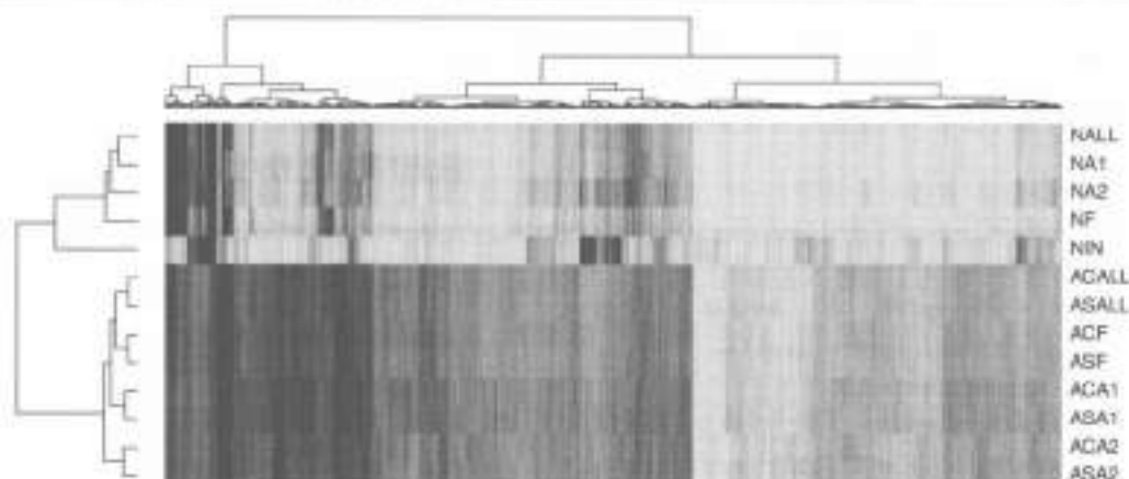
图 7.34 例5.1数据的热量图
