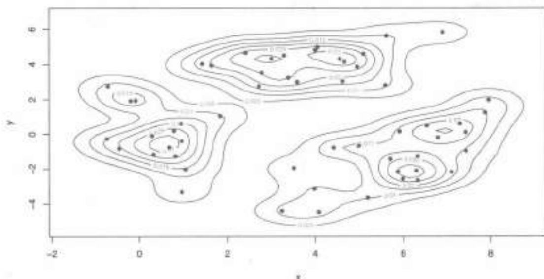
图 7.15 例7.4人造数据点云的非参数密度估计示意图
