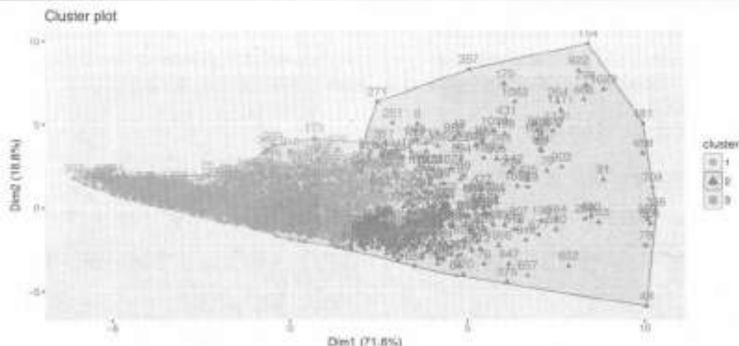
图 7.35 例5.1数据对观测值分层聚类(3类)的前两个主成分得分图
