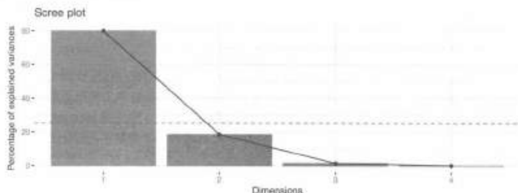
图 9.3 例9.1收入数据的收入和教育列联表的对应分析特征值的崖底碎石图
