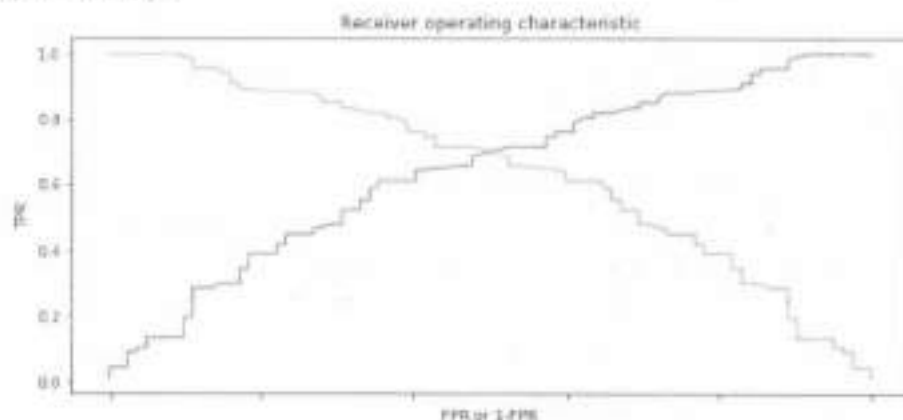
图 4.11 例4.2献血数据 Logistic 回归的 ROC 曲线 ( TPR 对 FPR ) 及曲线 ( TPR 对 1 - FPR )
