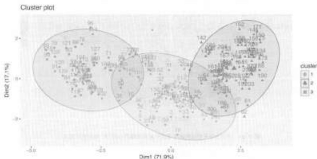
图 7.30 例7.6种子数据前两个主成分的观测值得分的 K 均值聚类情况
