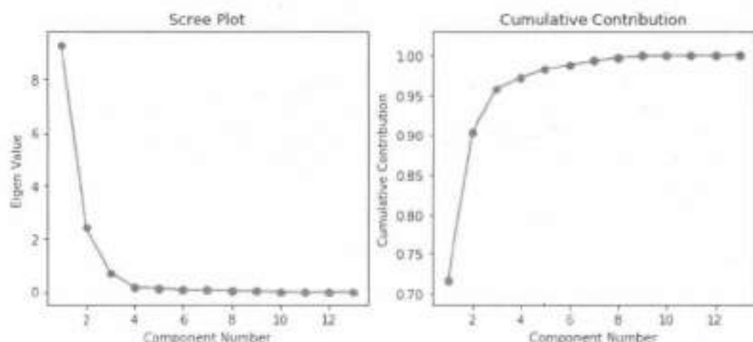
图 5.14 例5.1教师数据主成分分析的陡底碎石图
