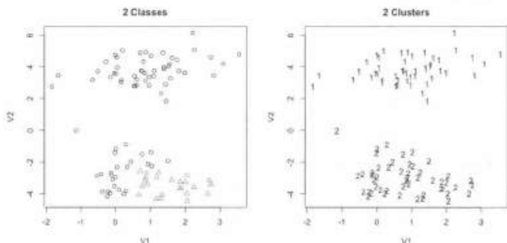
图 7.1 例 7.1 人造数据的分类 (左, 用圆圈和三角符号表示两类) 和聚类图 (右, 用 1 和 2 表示两类)
