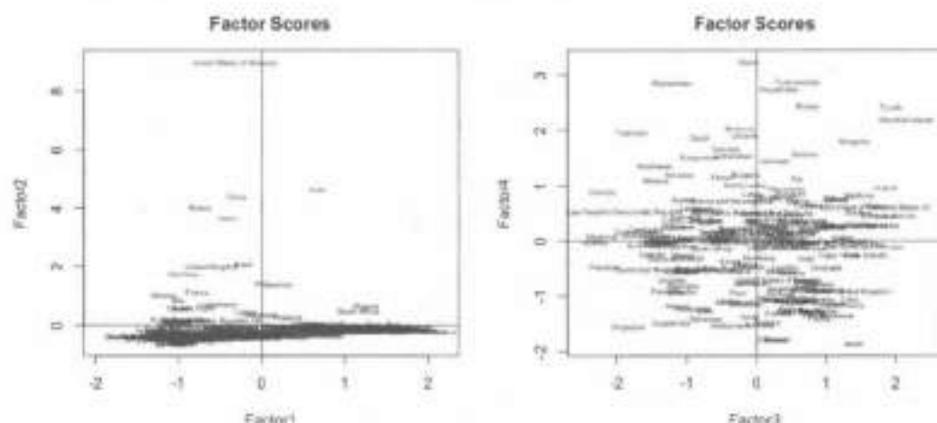
图 6.5 例 6.1 WHO 数据的因子得分图
