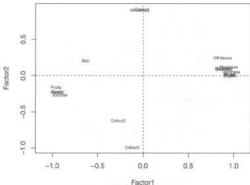
图 6.6 例6.2豌豆数据的因子分析的载荷图
