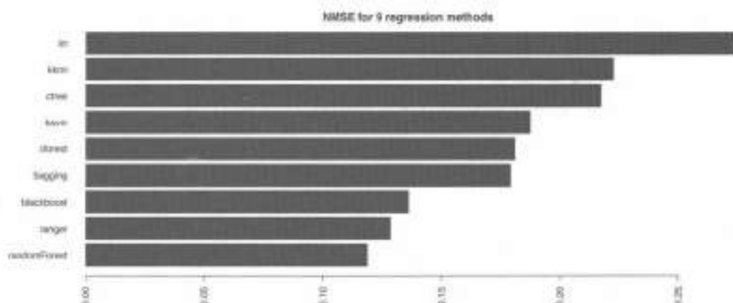
图 3.16 九种方法拟合例3.1波士顿住房数据的 NMSE 图
