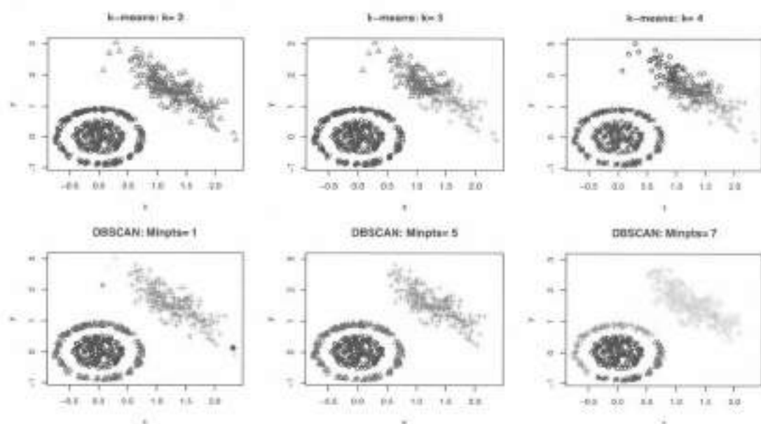
图 7.14 例7.5数据聚类: 对于不同 k 值 ( k = 2, 3, 4 ) 的 K 均值聚类及不同 Minpts 值 ( Minpts = 1, 5, 7 ) 的 DBSCAN 聚类结果, 不同的类用不同的符号表示
