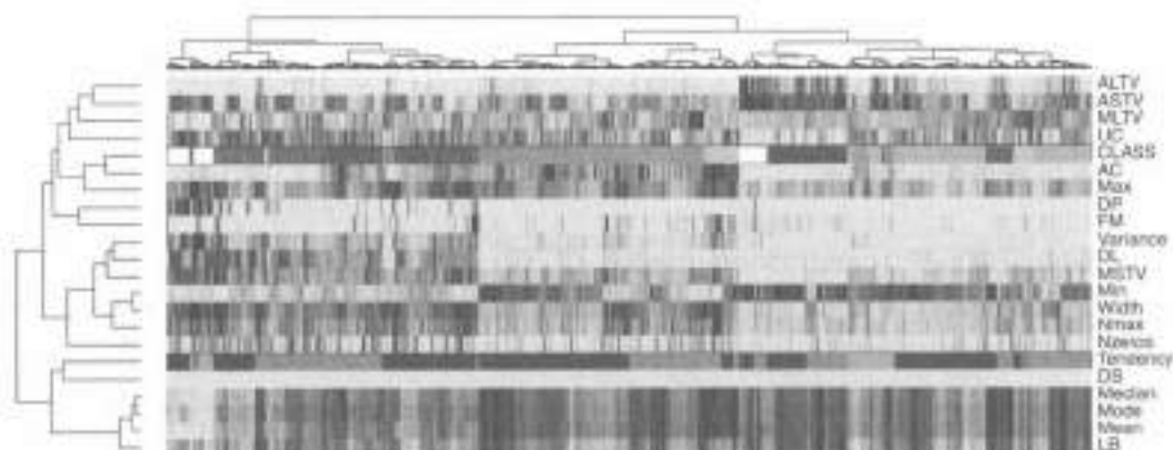
图 7.32 例7.7胎心宫缩监护数据的热量图
