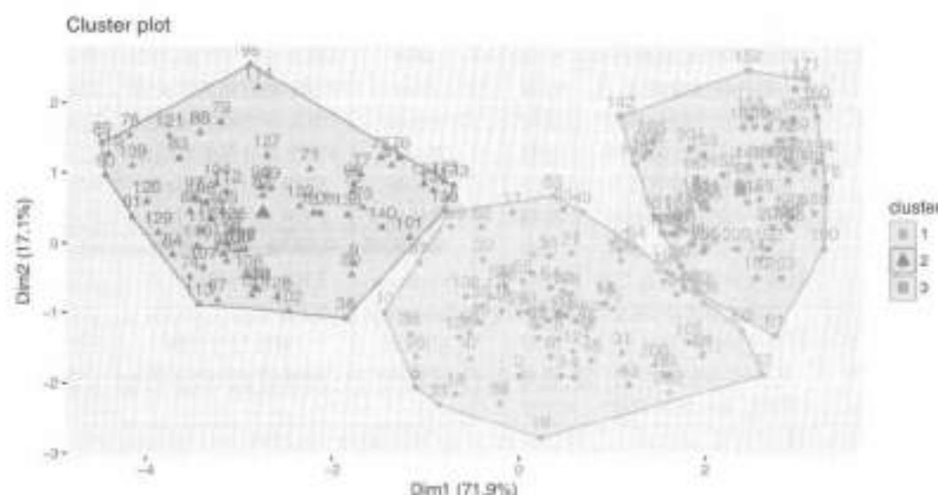
图 7.31 例7.6种子数据前两个主成分的观测值得分的分层 K 均值聚类情况
