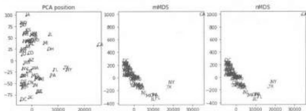
图 10.3 例10.2教育数据: 原始数据的主成分得分 (左)- mMDS(中) 及 nMDS(右)
