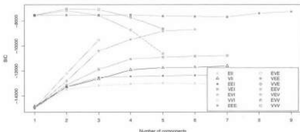
图 7.18 例6.1的基于模型聚类的 BIC 图
