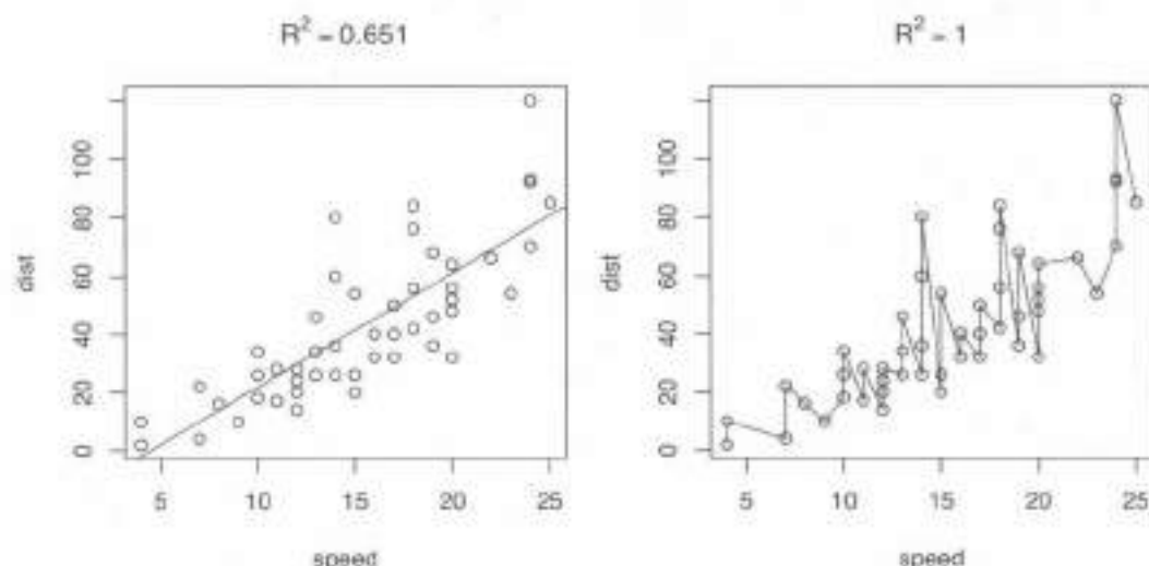
图 3.7 最小二乘回归和折线回归
