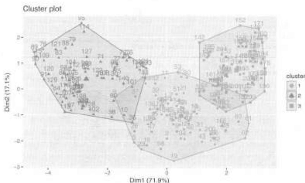
图 7.28 例7.6种子数据前两个主成分的观测值得分的K均值聚类情况
