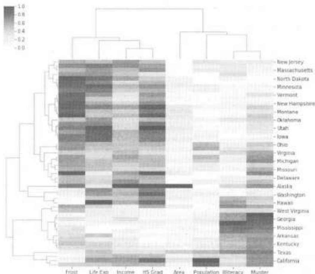
图 7.41 例7.2美国各州数据的热量图
