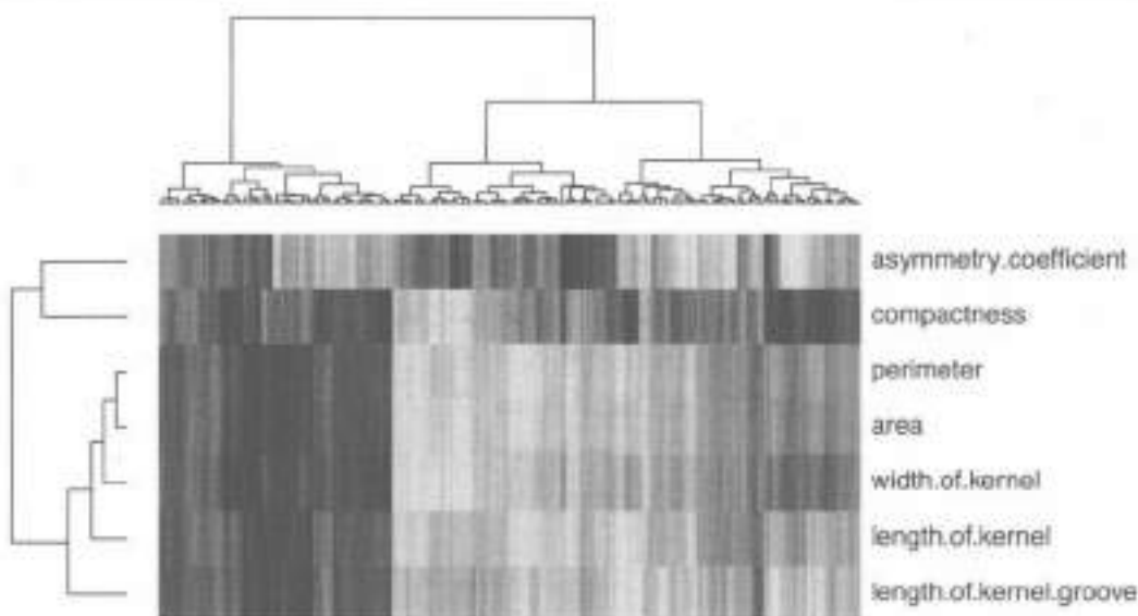
图 7.26 例7.6种子数据的热量图
