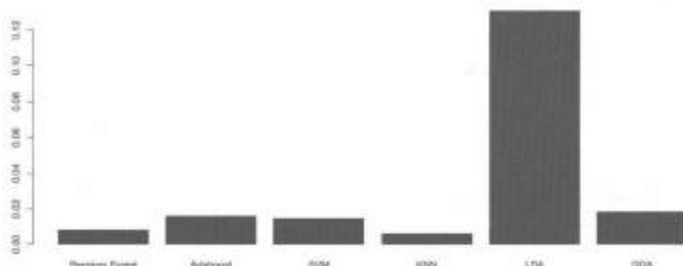
图 4.10 对例4.1数字笔迹识别数据分类的 6 种方法的测试集预测误判率
