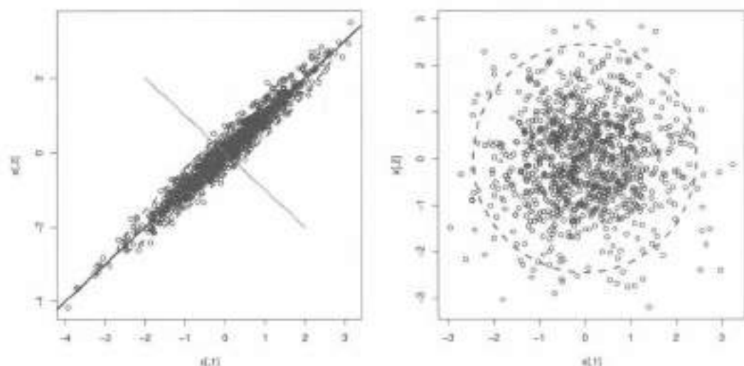
图 5.3 相关变量点云 (左) 及无关变量点云 (右)
