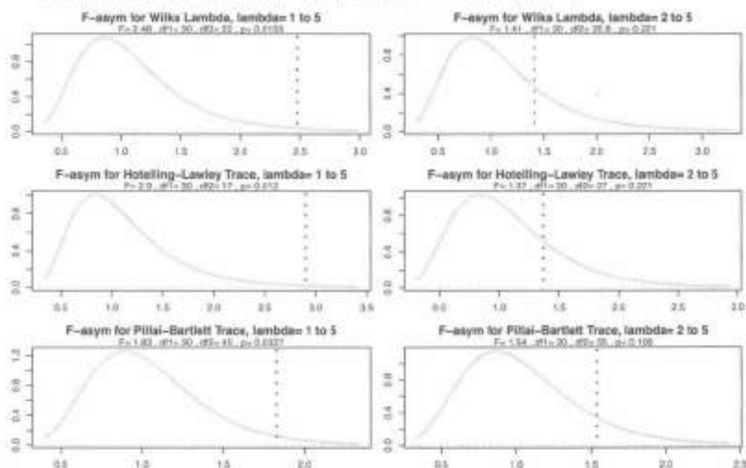
图 8.5 例 8.1 模拟数据的 Wilks、Hotelling、Pillai 检验分布图
