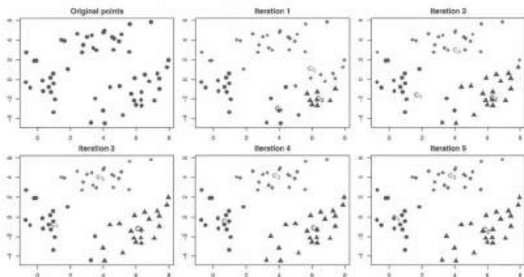
图 7.11 例7.4人造数据的 K 均值聚类 5 次迭代示意图 (每次迭代用实心的圆、菱形和三角形代表分的三类点)
