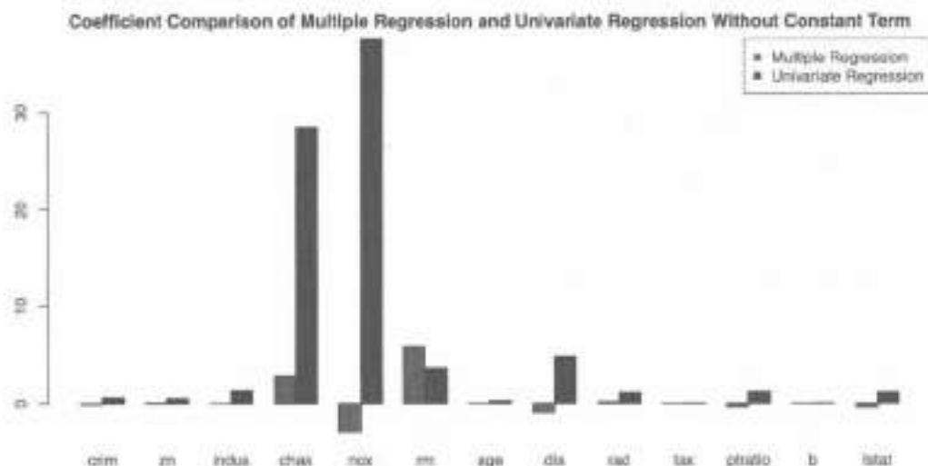
图 3.5 对例3.1波士顿住房数据做每个自变量的简单回归和多重回归系数估计的变化
