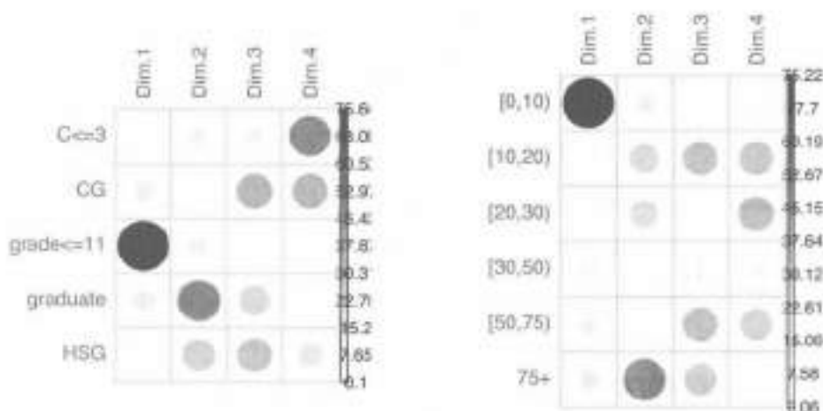
图 9.4 例9.1收入数据的收入和教育列联表的对应分析行列变量对各级的贡献
