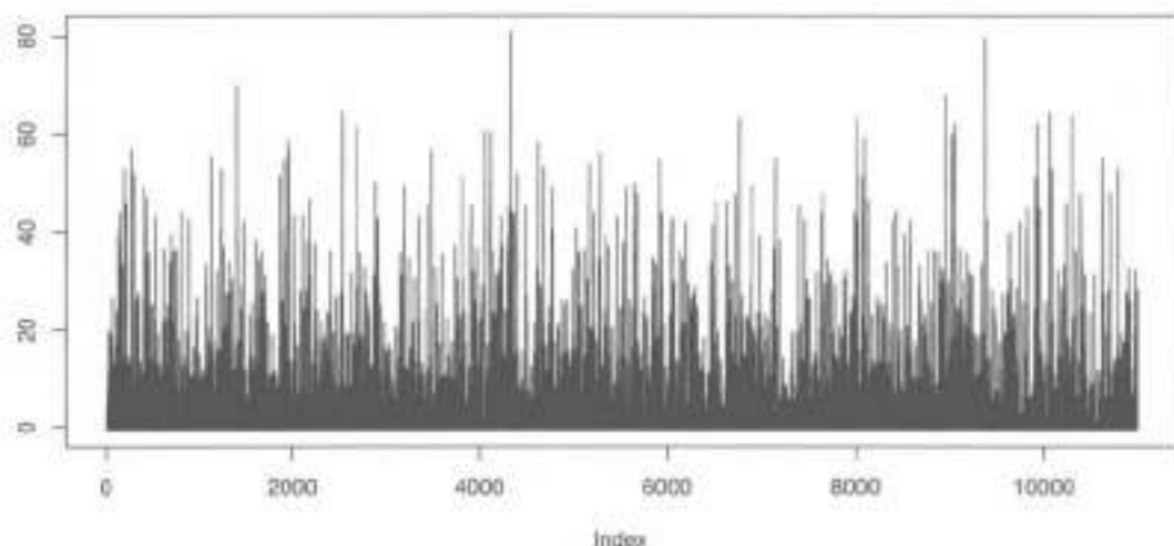
图 4.8 随机森林拟合例4.1数字笔迹识别数据的离群点图
