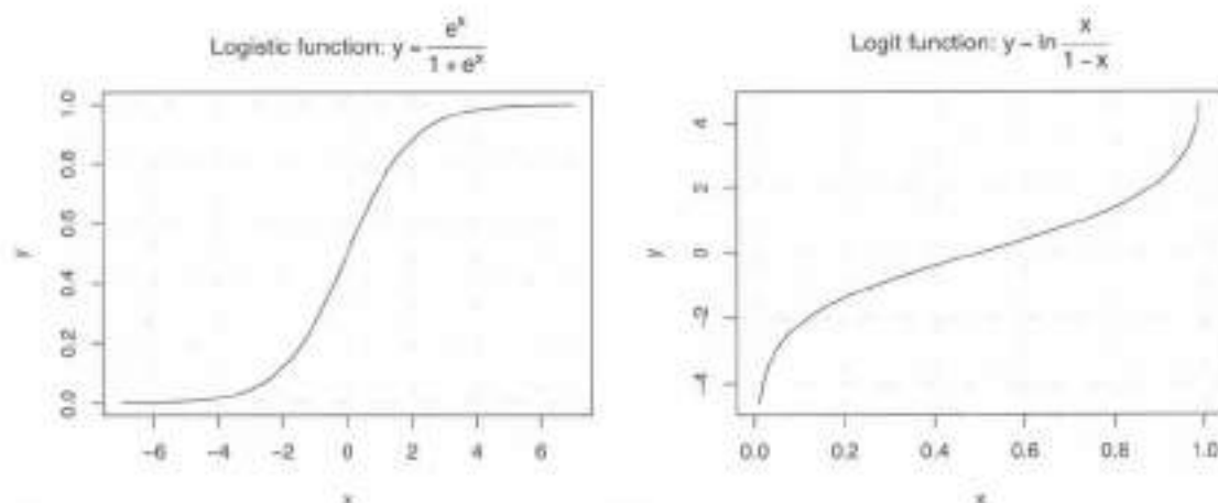
图 4.2 Logistic 函数 (左) 和 logit 函数 (右)
