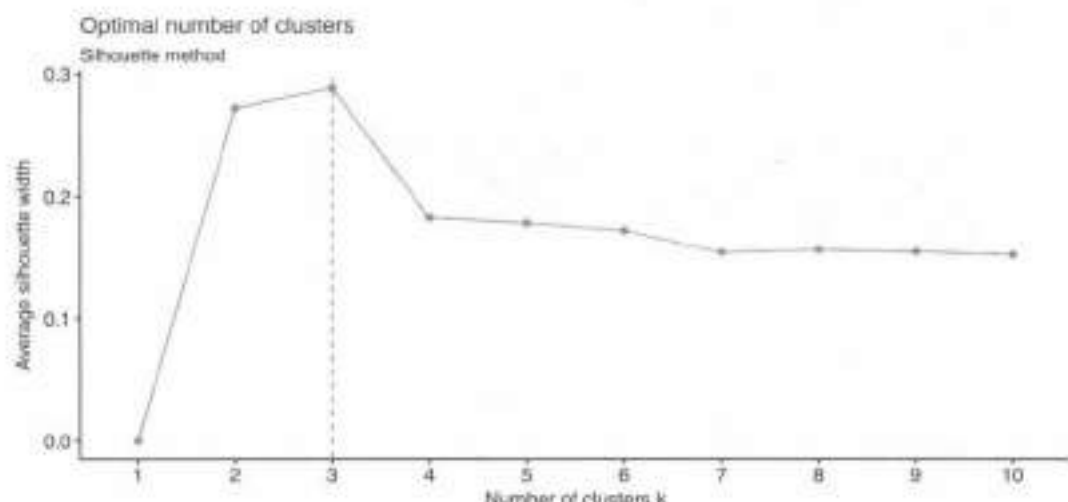
图 7.22 对例6.1利用不同聚类数目的平均轮廓宽度选择最优聚类个数 (3 个)
