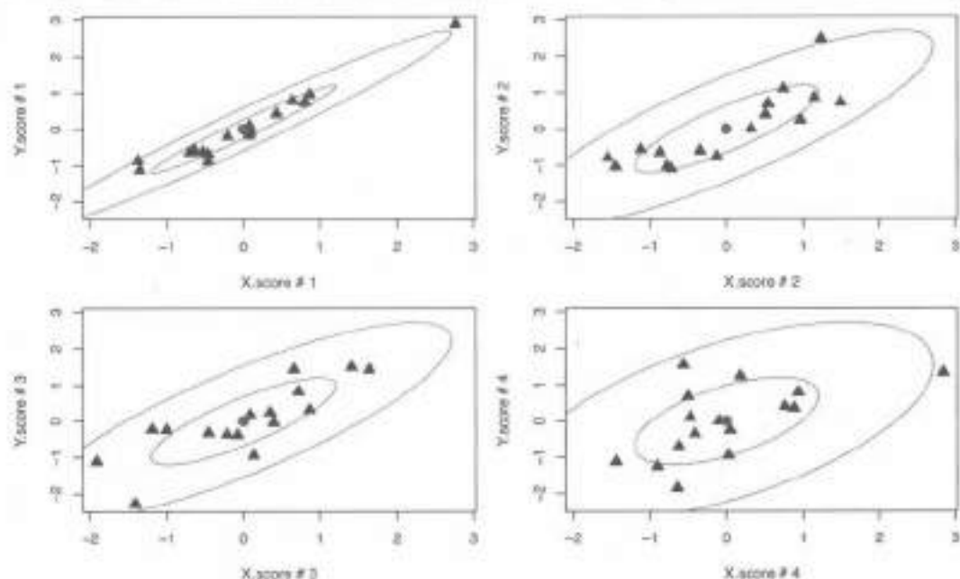
图 8.4 例8.1崖底油数据前4对典型相关变量记分点图
