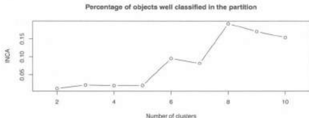
图 7.24 例6.1数据的 INCA 指数
