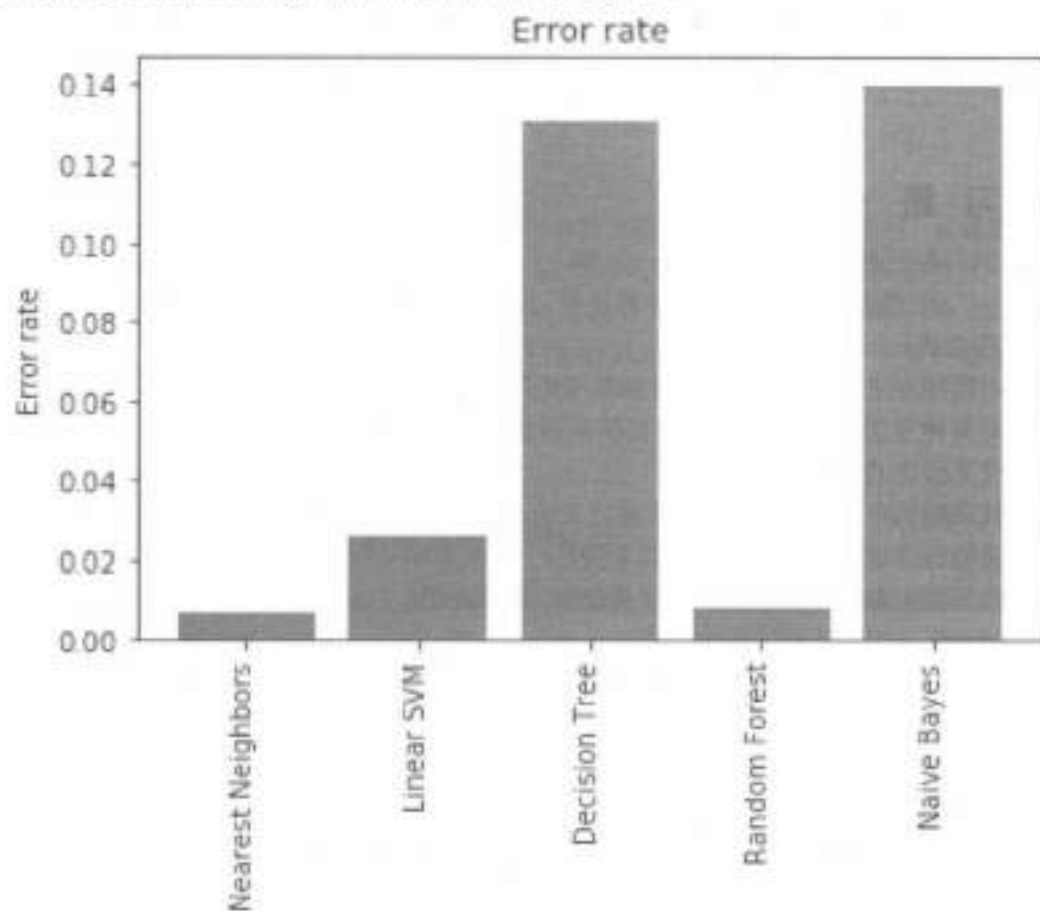
图 4.12 例4.1数字笔迹识别数据的 5 种机器学习方法分类 10 折交叉验证的误差率
